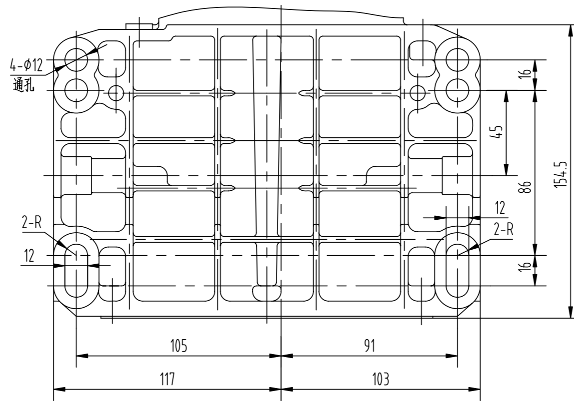
2V78F-2 安装尺寸图
