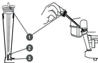
Рис. 20. Крышка-щуп маслозаливной горловины
