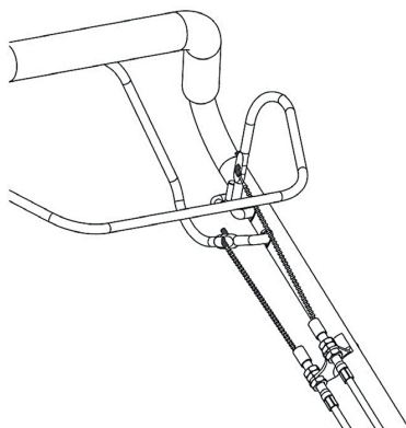
Рис.3 Правильная установка тросов
