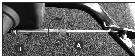
Рис.23 Регулировка троса привода хода
