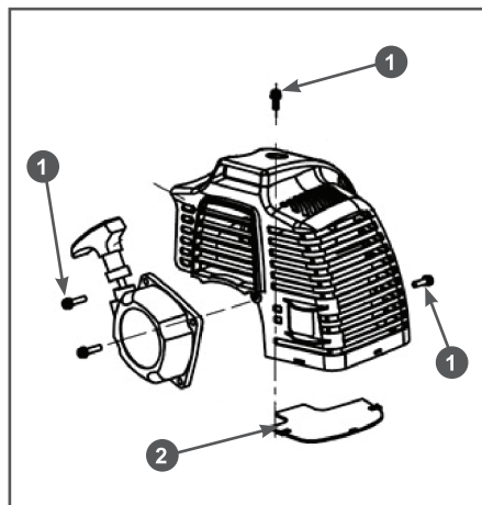
Рис. 12 Очистка охлаждающих ребер цилиндра
