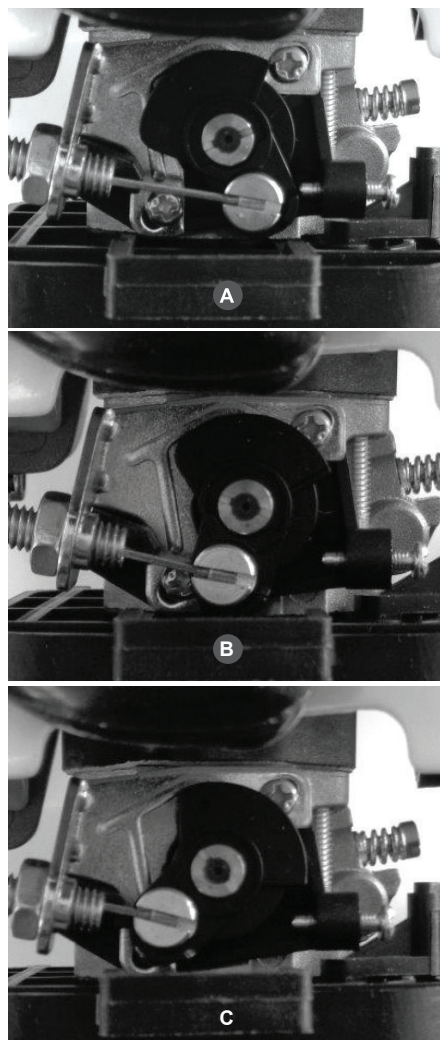
Рис. 4 Положение кронштейна дроссельной заслонки
