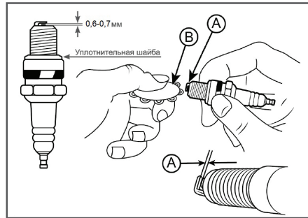
Рис. 11 Проверка зазора между электродами
