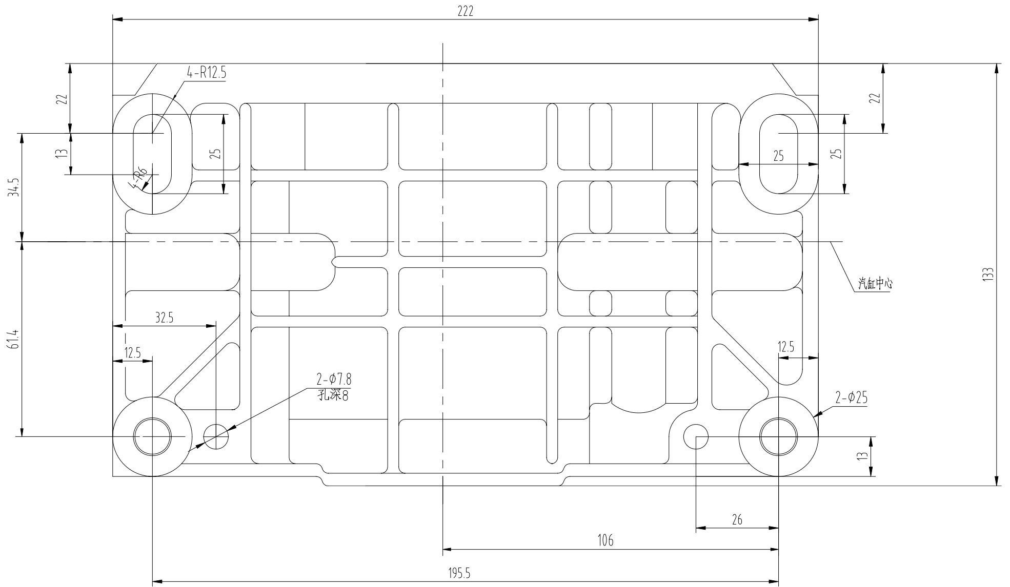
173F/177F 底板安装尺寸
