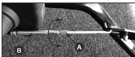
Рис.23 Регулировка троса привода хода
