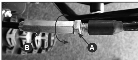
Рис.30 Регулировка троса включения шнека
