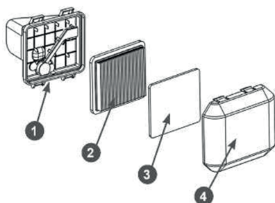
Рис. 24. Обслуживание воздушного фильтра
