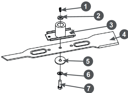
Рис. 28. Установка ножа
