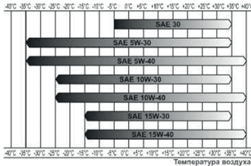
Рис. 14. Определение вязкости масла
