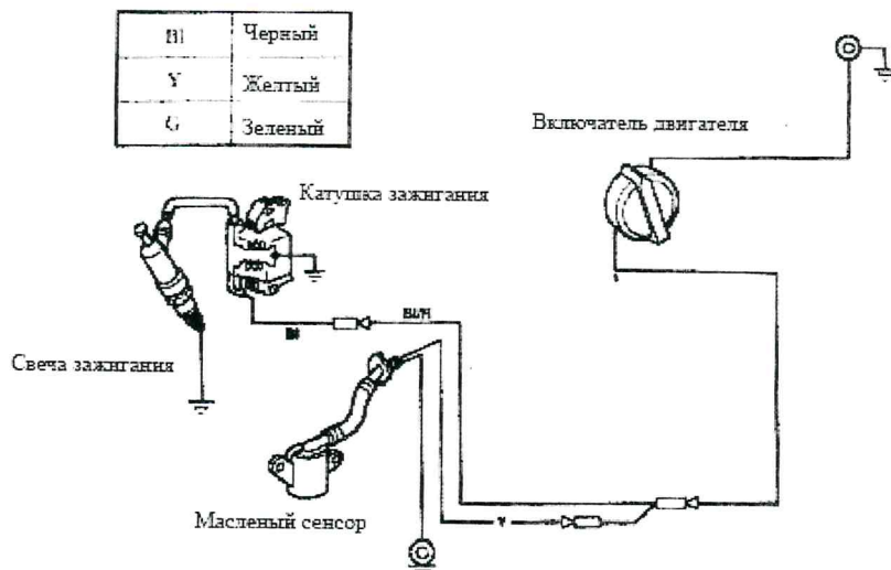
Электродиаграмма
