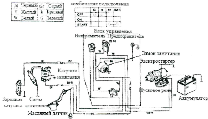
Электродиаграмма
